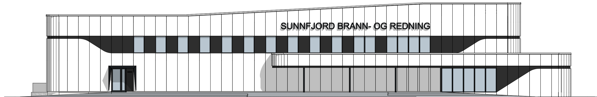
1:200 Fasade Sør
