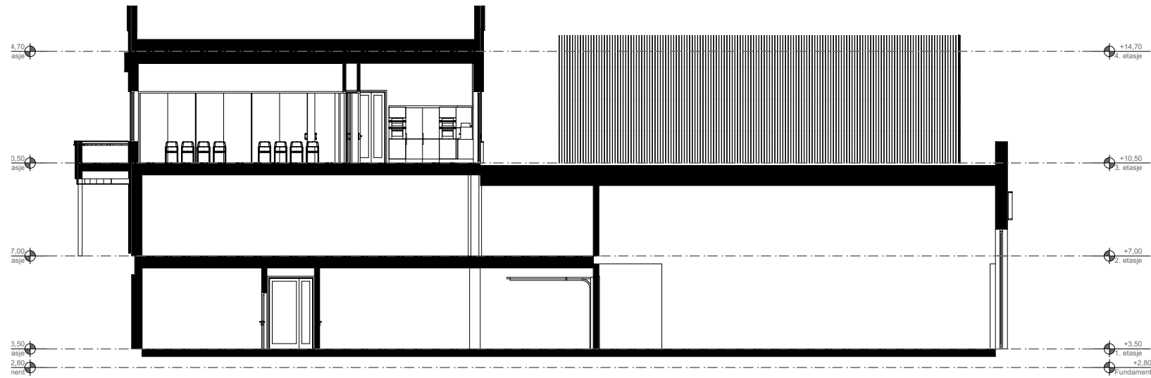
1:200 Snitt A
