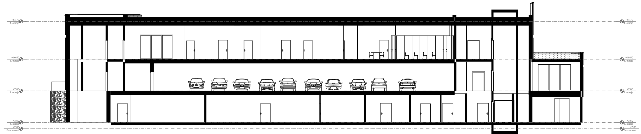
1:200 Snitt 1
