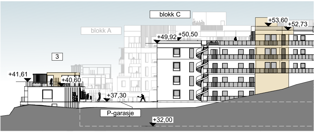
1:500 Fasade SØ Småhus blokk C
