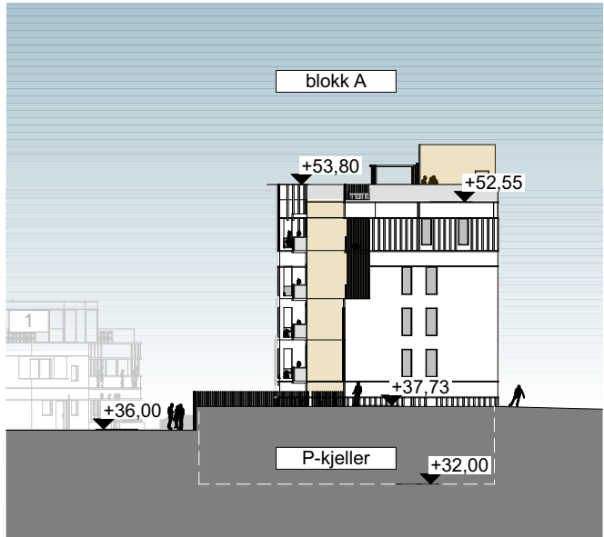
1:500 Fasade Ø
