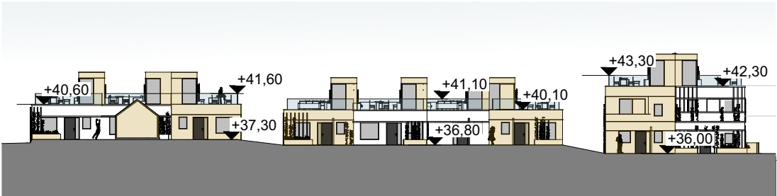
1:500 Fasade NØ Småhus
