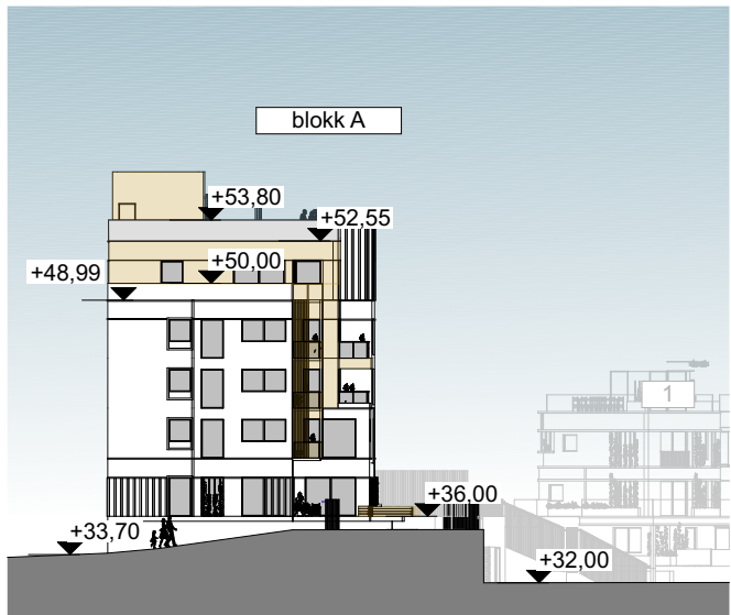
1:500 Fasade V
