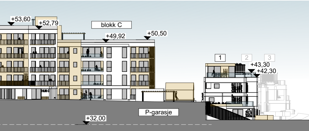
1:500 Fasade NV Blokk C Småhus
