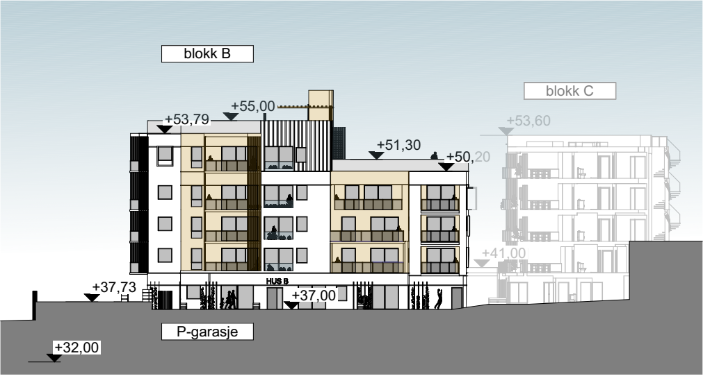
1:500 Fasade S
