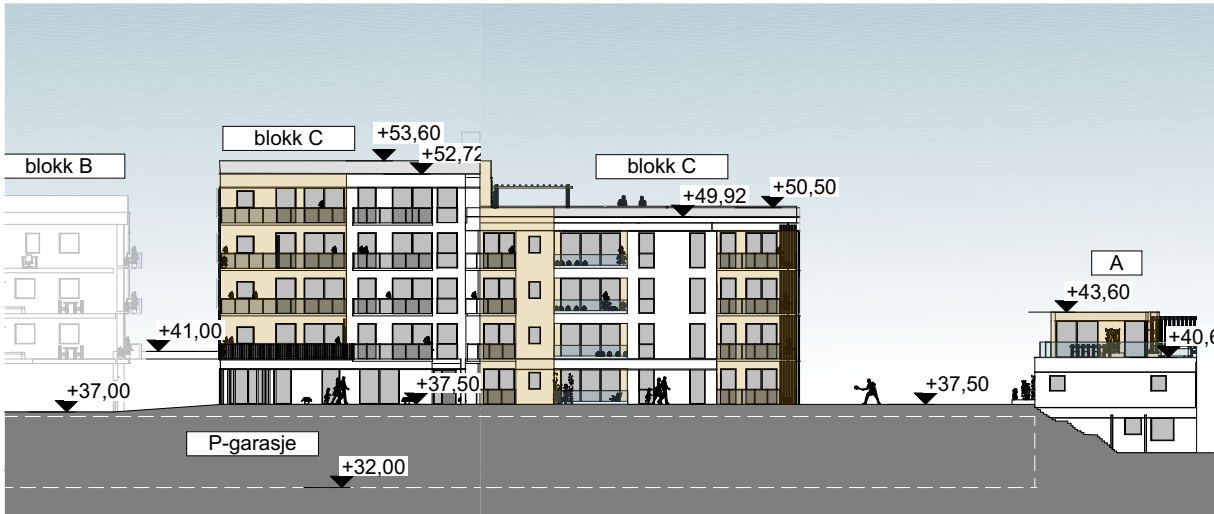
1:500 Fasade V
