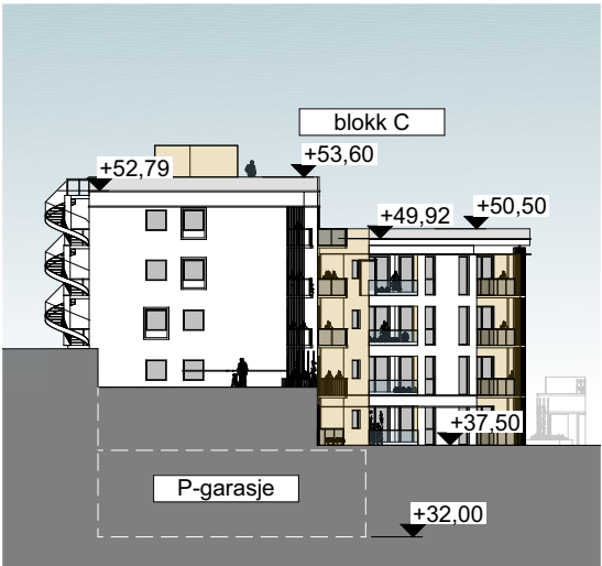
1:500 Fasade N
