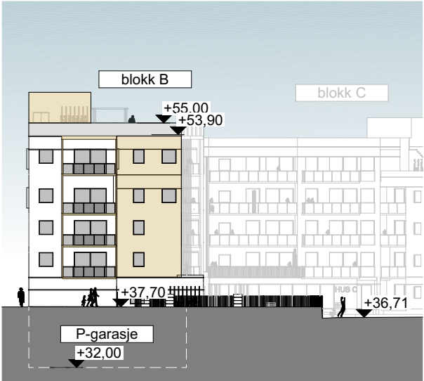
1:500 Fasade V
