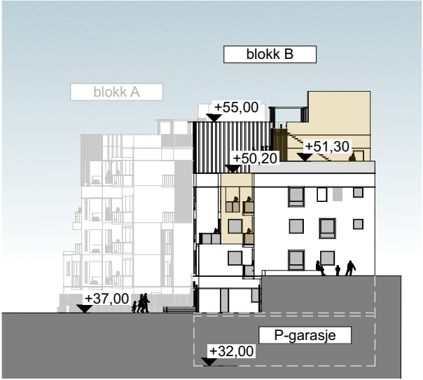
1:500 Fasade Ø
