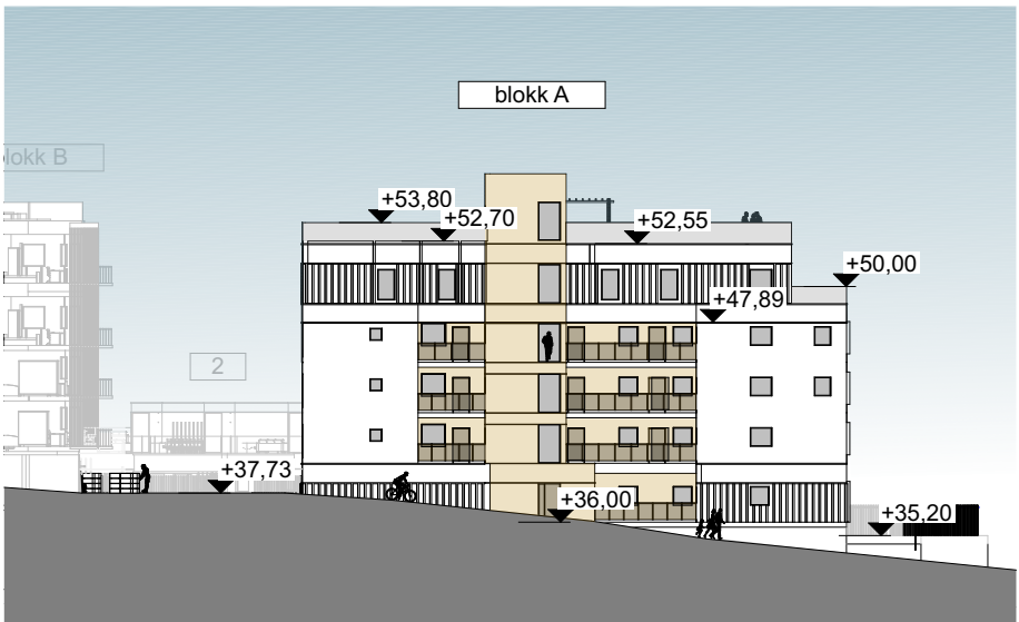
1:500 Fasade N
