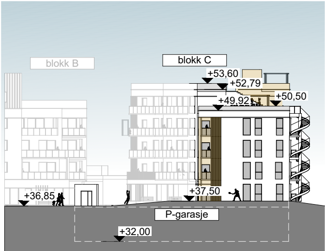
1:500 Fasade S
