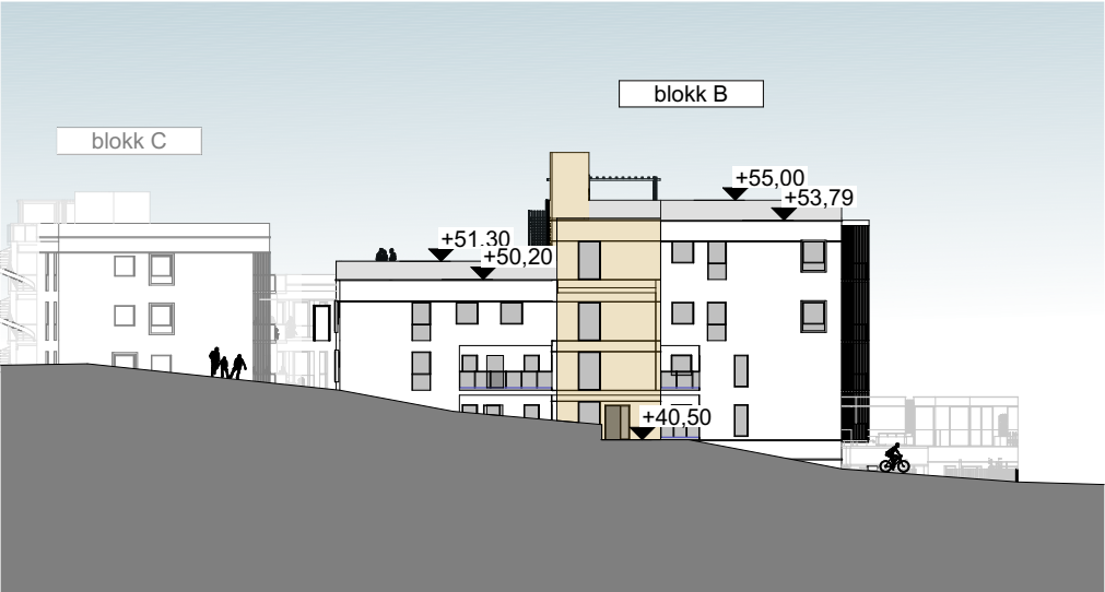
1:500 Fasade N
