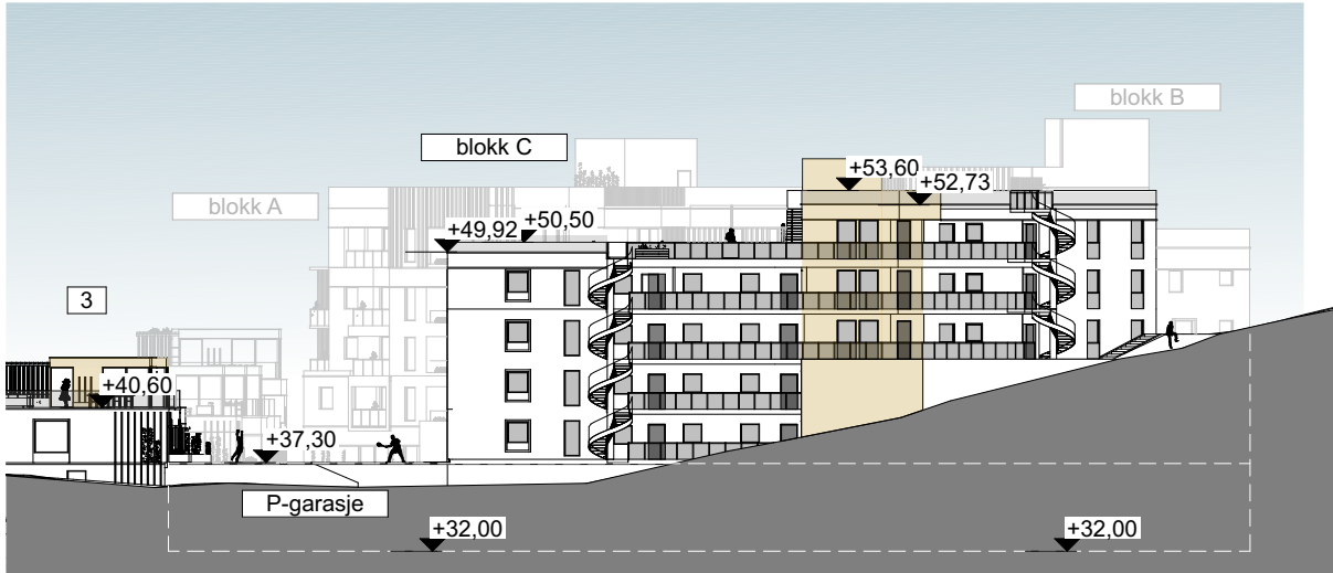
1:500 Fasade SØ Småhus blokk C
