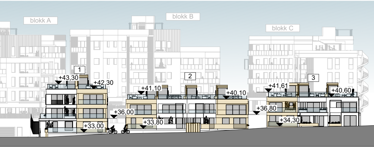
1:500 Fasade SV Småhus
